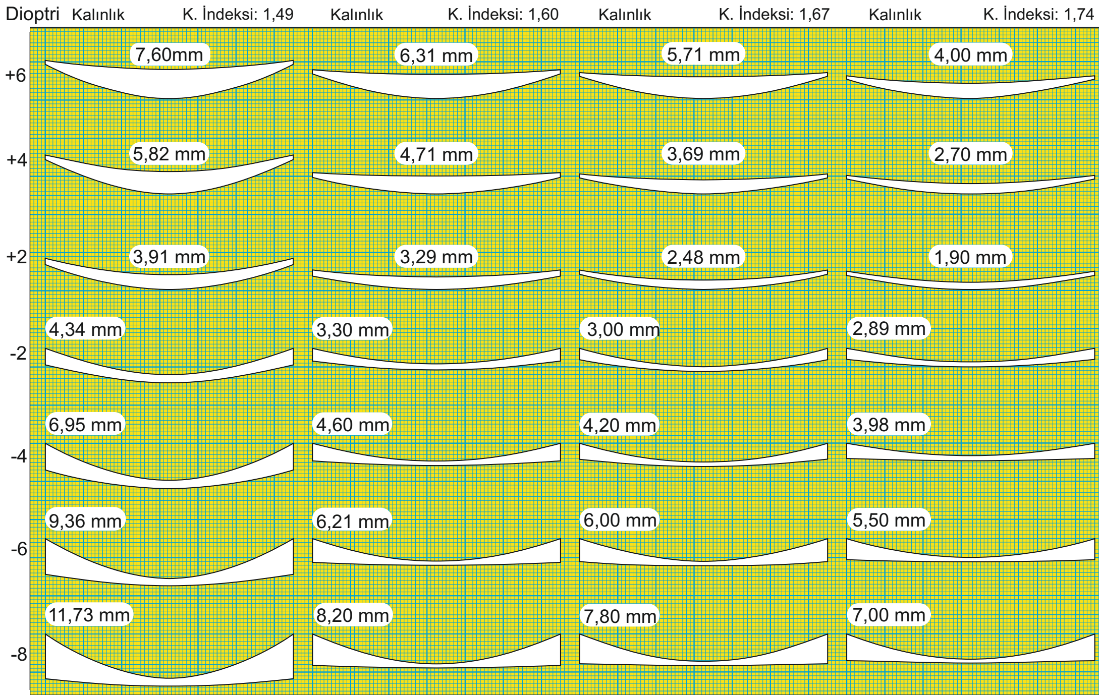
Şekil: Farklı dioptriler için farklı hammadde kırma indeksleri ile optik camların incelmesini gösteren şematik çizim. Kılavuz niteliğindedir, cam şekli reçete ve çerçeve seçimine bağlı olarak değişebilir. Farklı bir cam üretici kataloğundan esinlenerek, Dr. Ercan Mensiz tarafından çizilmiştir. Serbestçe dağıtılabilir. www.amansees.com
